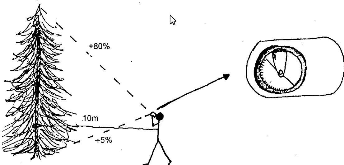
Hình 6.1.4: Thước đo độ cao (thước Bumleiss)
