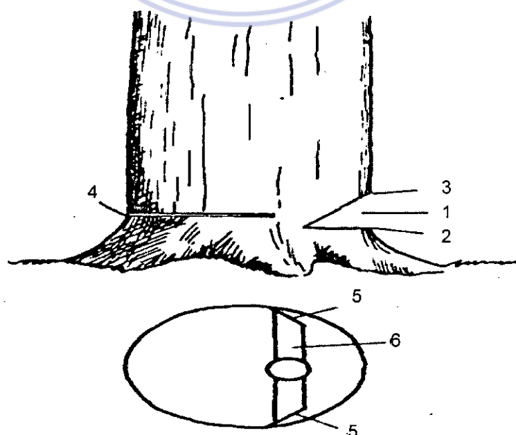
Hình 6.2.5: Thao tác mở miệng từ hai bên
